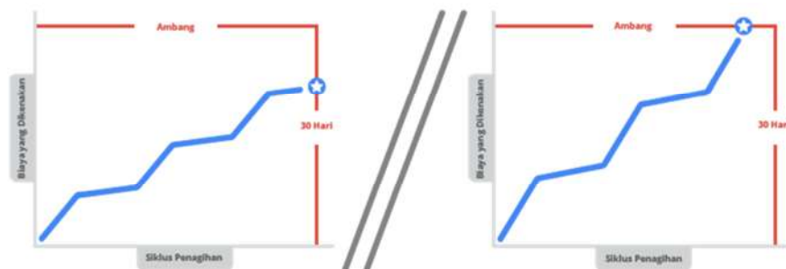
Gambar 6.17 Ilustrasi penagihan
