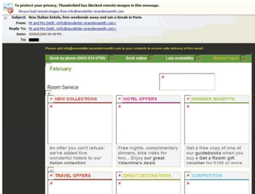
Gambar 5.14 Pemblokiran Gambar.
